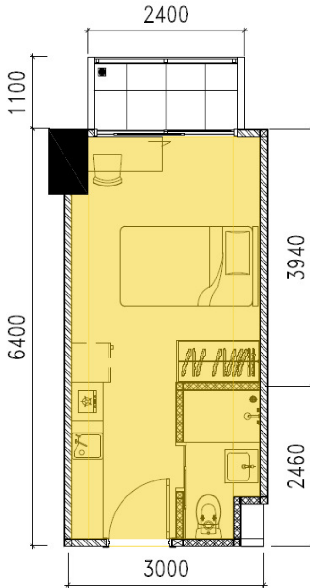
UNIT STA Semigross = 27,82 m 2
